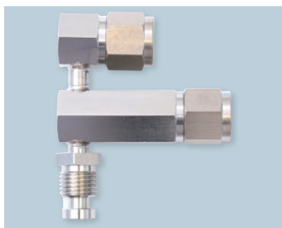
■ 2段エルボユニオン 溶接タイプ
